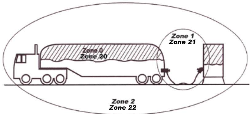
Tegningen viser et eksempel på Zone-inndeling. Gass: Zone 0, 1 og 2. Støv: Zone 20, 21 og 22.
